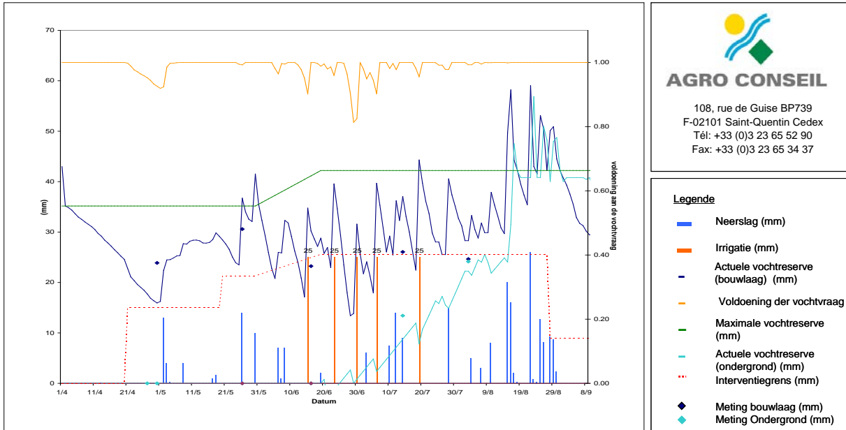
Vochtbalans Jos Van Sambeek, Reusel
